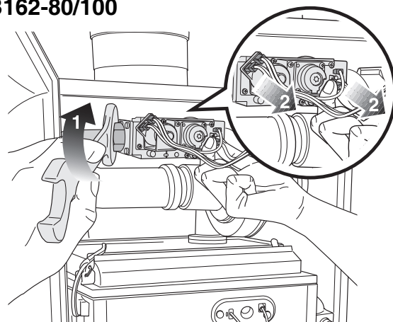
Fig. 100 Tilslutningerne på gasarmaturet løsnes
