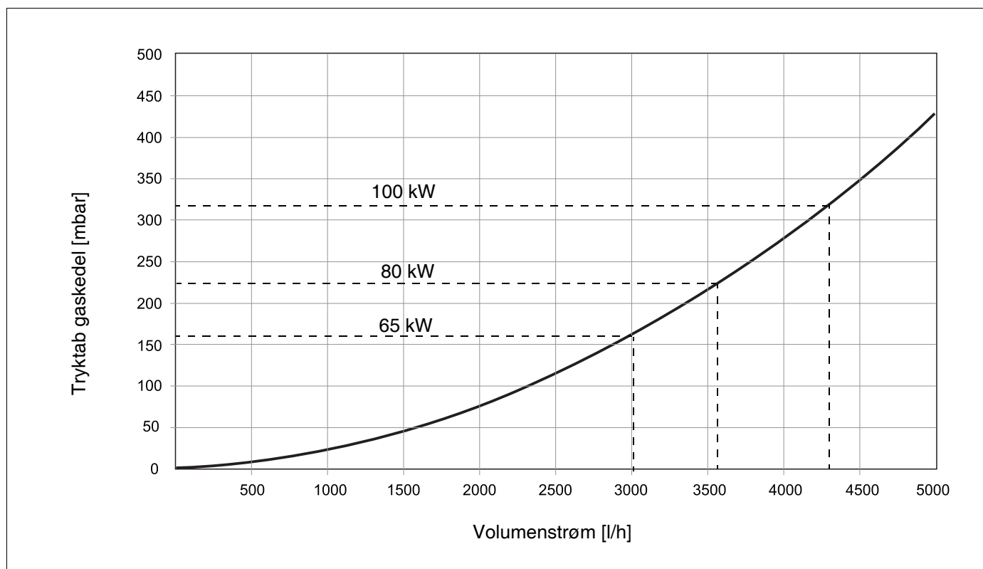
Fig. 120 Tryktab gaskedel
