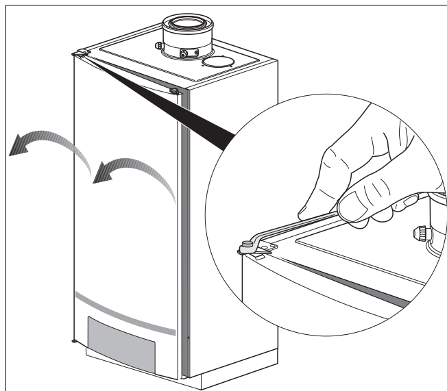
Fig. 99 Afmontering af kedeldøren
