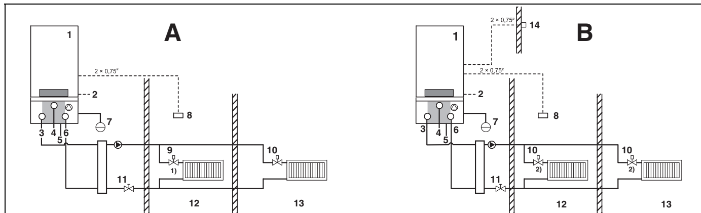
Fig. 7 Anlægseksempler A: og rumtemperaturstyring B: og vejrkompensering
