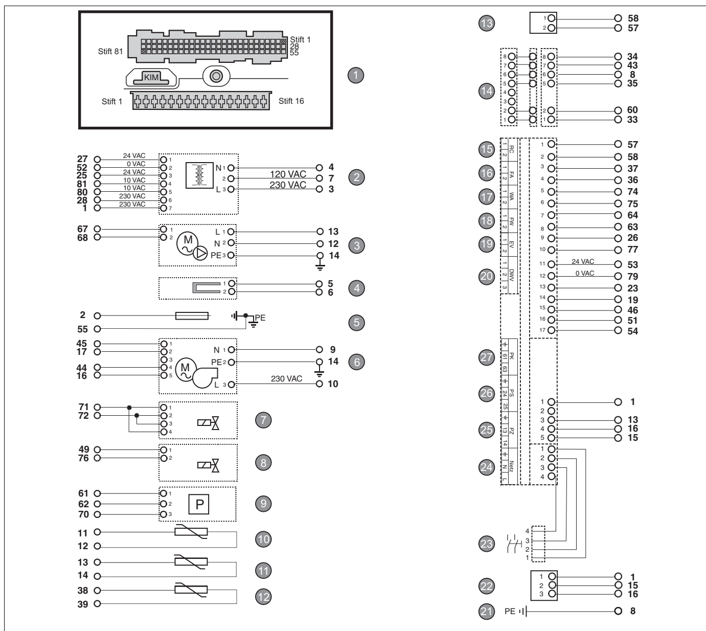
Fig. 122 Eldiagram Logamax plus GB162-65/80/100
