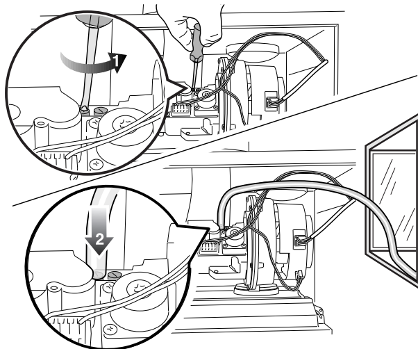
Fig. 74 Gashanen lukkes
