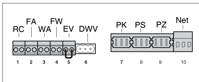
Fig. 27 Klemmerækker
