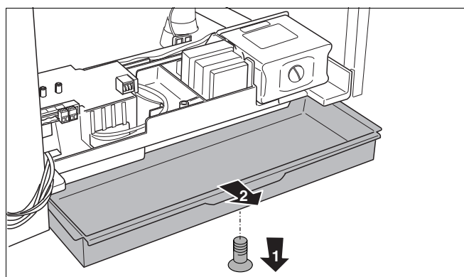
Fig. 44 Åbning af skuffen
