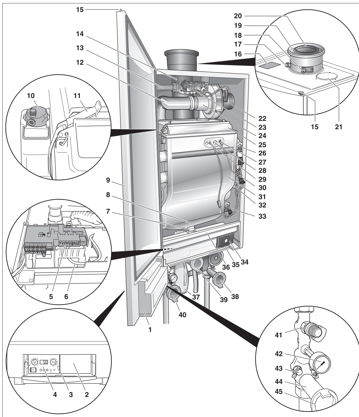
Fig. 1 Logamax plus GB162-65/80/100 med tilslutningsgruppe
