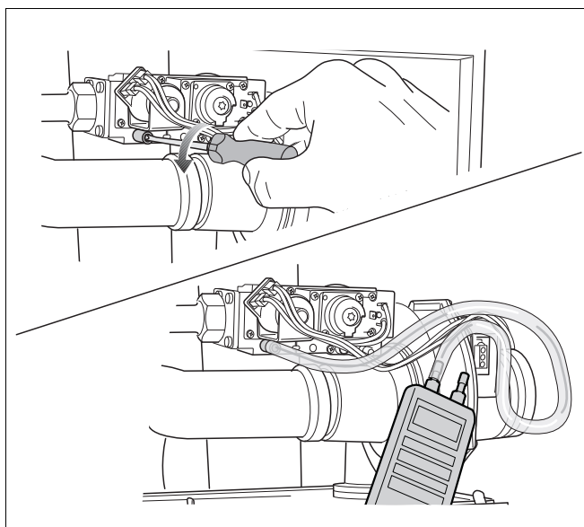
Fig. 98 Kontrol af gasarmaturet for indre tæthed
