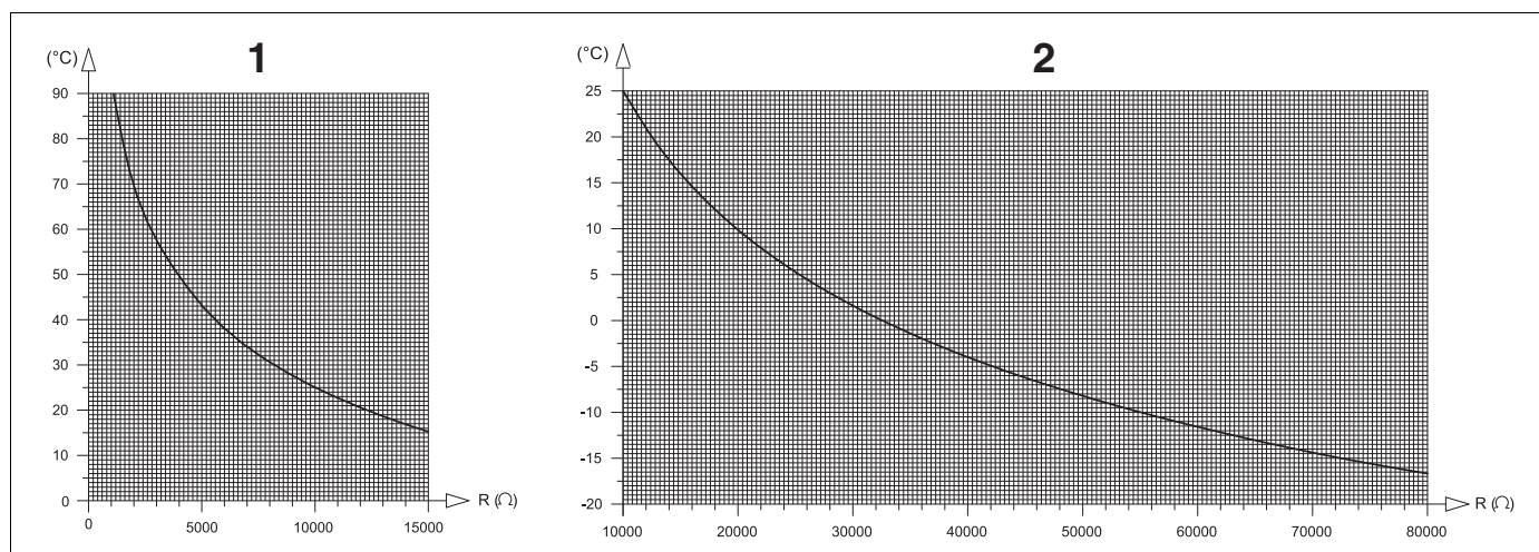
Fig. 121 Modstandskarakteristik NTC-føler
