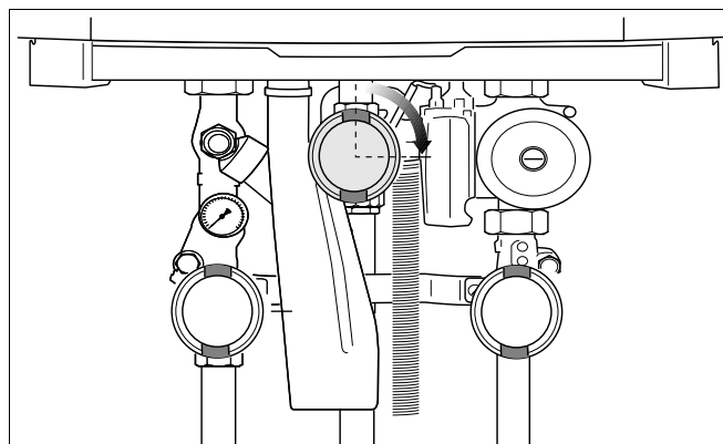
Fig. 74 Gashanen lukkes
